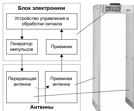
Структурная схема металлодетектора
