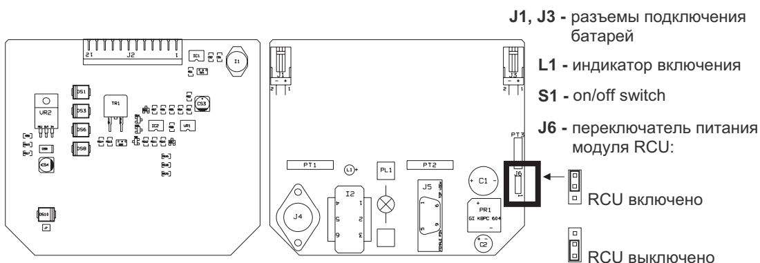
Плата ALP с устройством зарядки батарей
