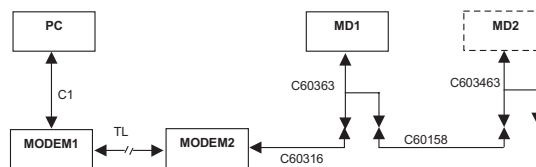
Схема подключения к телефонной линии: PC - компьютер; MD1, MD2 - металлодетекторы; с1 - модемный кабель; TL - телефонная линия.
