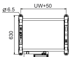
Размещение отверстий для крепления к полу (UW=680/760 мм).
