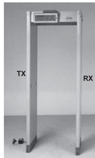
Передающая антенна TX с левой стороны
