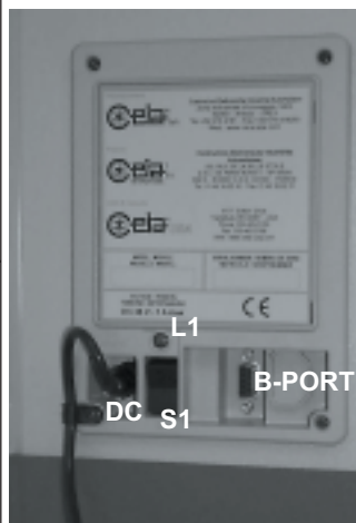
Нижняя панель соединений.
