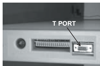
Разъемы для подключения последовательного порта на металлодетекторе.
