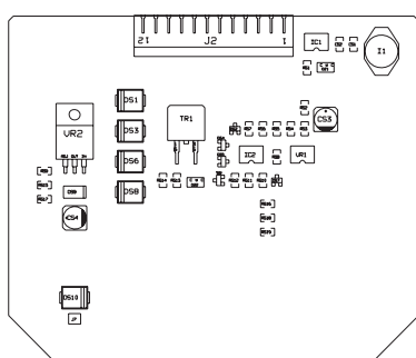
Плата ALP с устройством зарядки батарей
